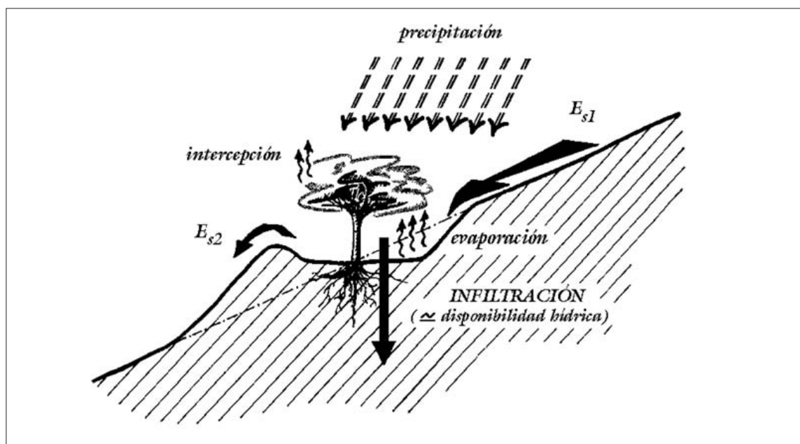
Figura 2 Componentes principales del balance hídrico local (MARTÍNEZ DE AZAGRA 1996).
