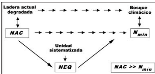
Figura 4 Serie progresiva del número de curva (MARTÍNEZ DE AZAGRA 1996). NAC = Número de curva de la ladera actual degradada; N min = Número de curva final en la ladera restaurada; NEQ = Número de curva equivalente de la unidad sistematizada.
