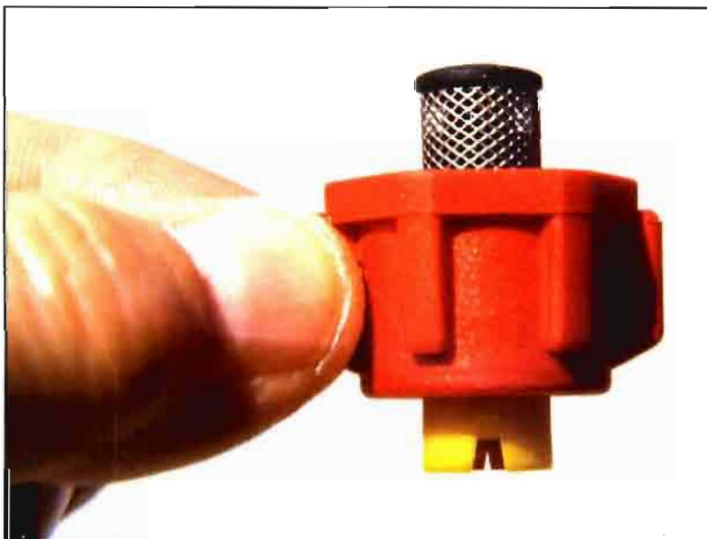
Un elemento importantísimo es la boquilla, de cuya calidad depende un uniforme reparto de la mezcla herbicida sobre la superficie tratada. Dotar a la boquilla de un adecuado equipo de filtrado es indispensable para evitar obturaciones, lo que influye negativamente en los resultados.
