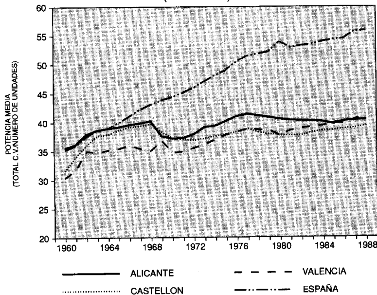
GRAFICO 3 EVOLUCION DE LA POTENCIA MEDIA DE LOS TRACTORES EN EL PAIS VALENCIANO (1960-1988)
