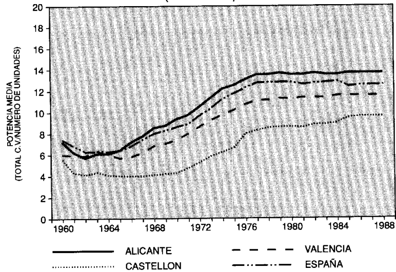
GRAFICO 4 EVOLUCION DE LA POTENCIA MEDIA DE LOS MOTOCULTORES EN EL PAIS VALENCIANO (1960-1988)
