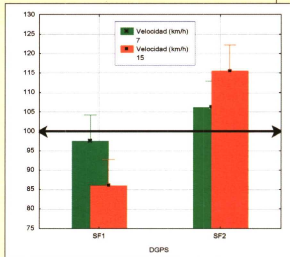
FIGURA 6. Valores medios de las distancias entre pasadas por distinta velocidad y nivel de precisión de señal en las trayectorias circulares.
