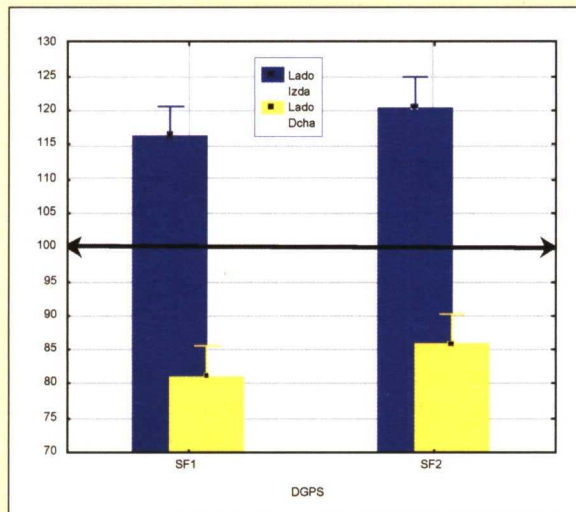
FIGURA 5. Valores medios de las distancias entre pasadas medidos alternativamente (lado izquierdo, lado derecho) en las trayectorias lineales.
