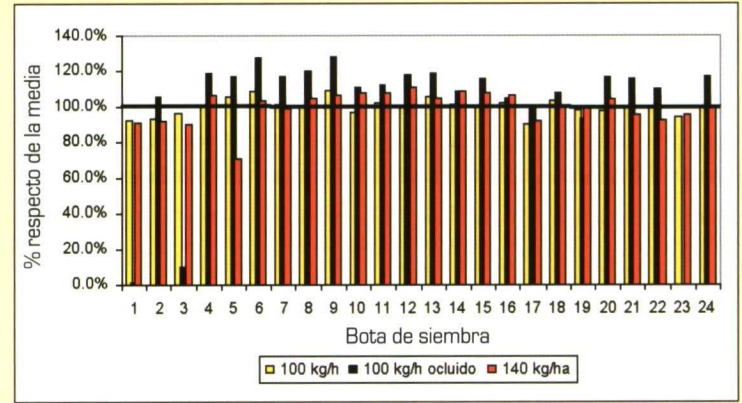
Figura 4. Distribución transversal de la semilla obtenida en los distintos tubos de descarga en el ensayo estático con guisante.
