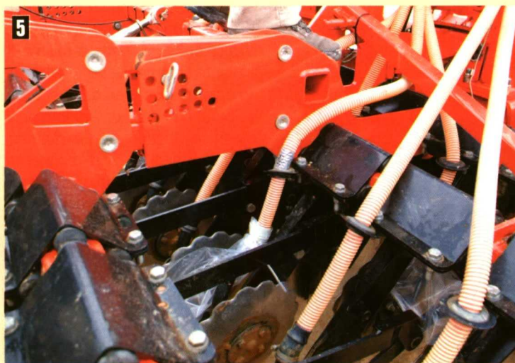
Dispositivo para la regulación de la profundidad de siembra.
