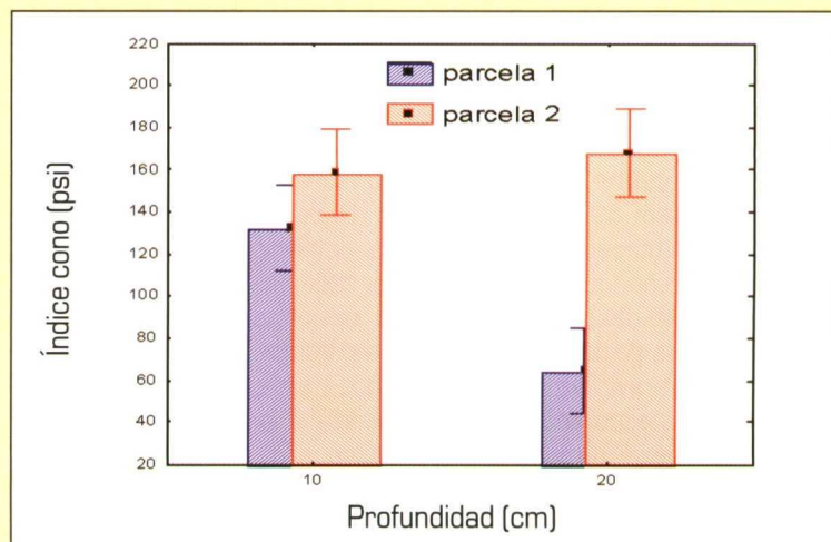
Figura 2. Determinación de índice de cono para evaluar la resistencia a la penetración del suelo en ambas parcelas.
