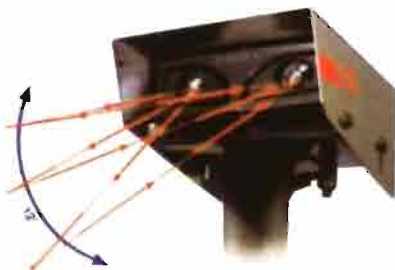
Derecha, arriba. El autoguiado Autotrack de John Deere se basa en GPS, igual que el de sus tractores.
