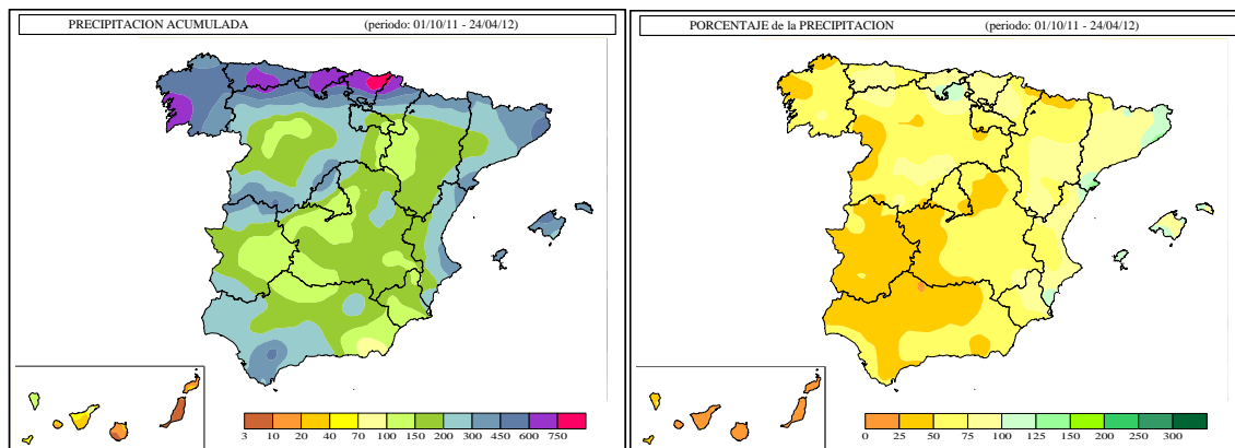
Figura 1. Precipitación acumulada en mm y porcentaje de precipitación (media 1970/2000) a 24 de abril de 2012 (Fuente: AEMET)
