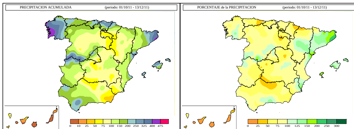
Figura 1. Precipitación acumulada y porcentaje de precipitación al 13 de diciembre de 2011 (Fuente: AEMET)
