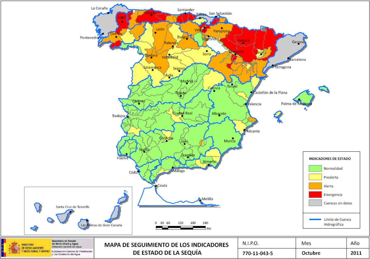
Figura 10. Mapa de seguimiento de la sequía (Octubre 2011) (Fuente: Observatorio Nacional de la Sequía)
