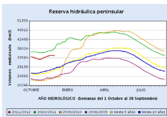
Figura 2. Reserva hidráulica total – semana del 30 de noviembre al 6 de diciembre de 2011 (Fuente: Boletín Hidrológico)
