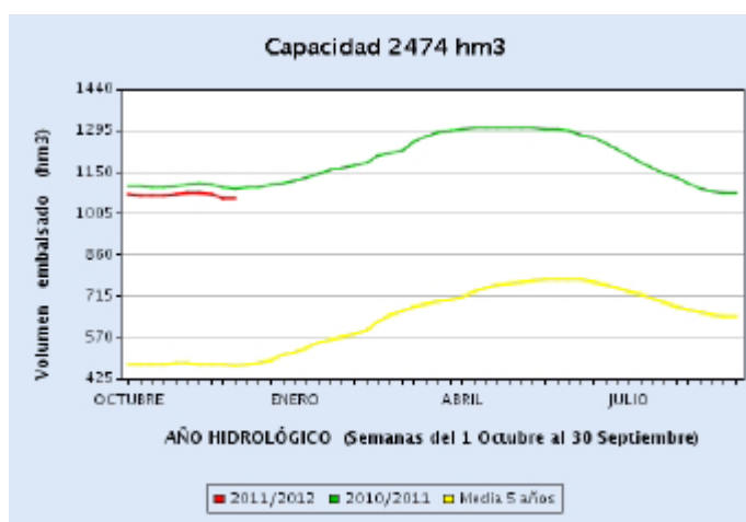
Figura 7. Volumen embalsado en la cabecera del Tajo a 6 de diciembre de 2011 (Fuente: Boletín Hidrológico)
