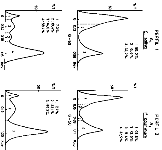
Fig. 4. Curvas de filtración a través de Sephadex G-50 y G-100 de los ácidos húmicos (porcentajes de las diferentes fracciones).
