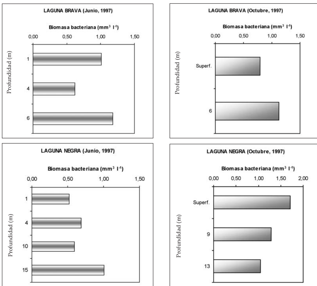
Figura 2 - Distribución vertical de la biomasa bacteriana en las lagunas Brava y Negra en junio y octubre de 1997. Figure 2 - Vertical profiles of bacterial biomass in Brava and Negra lakes in June and October 1997.
