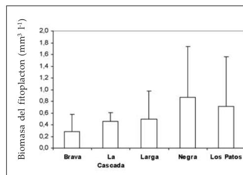
Figura 6 - Promedios y desviaciones típicas de la biomasa fitoplanctónica superficial, excluyendo el picoplancton, en las lagunas de Neila.
