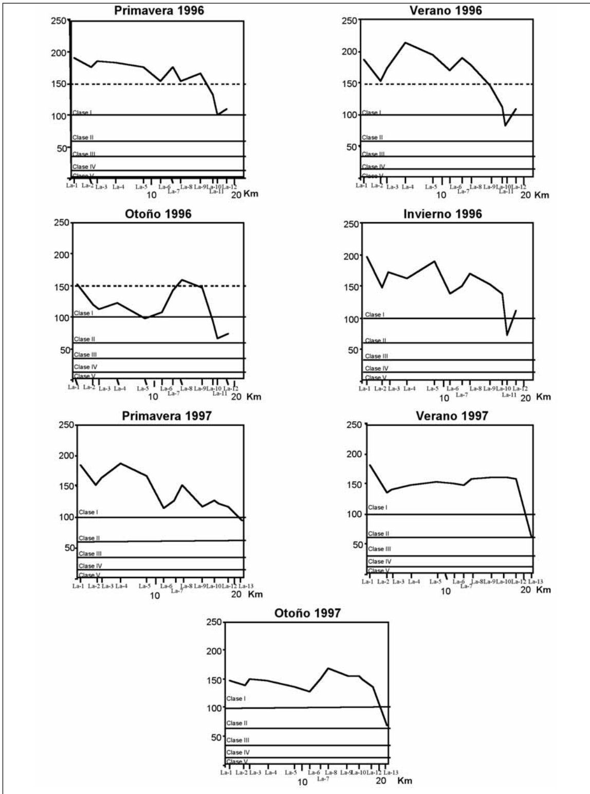
Figura 2 - Valores del índice BMWP' en el río Larraun (1996-1997).
