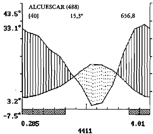
Fig. 1. Climodiagrama.
