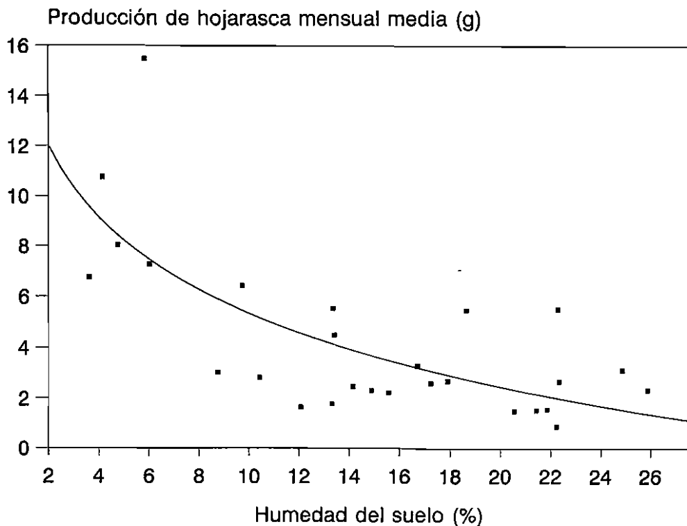
Fig. 3. Regresión logarítmica entre los valores mensuales de humedad edáfica y la producción de hojarasca de Rosmarinus officinalis . p < 0.0001 .
