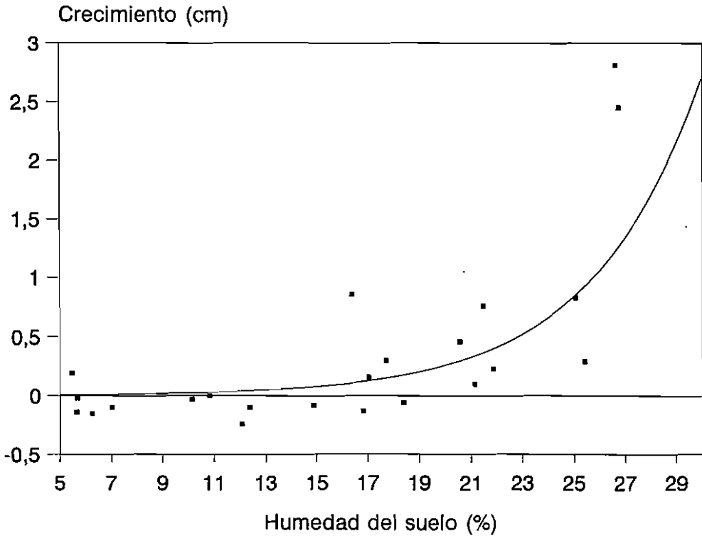
Fig. 2. Regresión exponencial entre los valores mensuales de humedad edáfica con dos meses de retardo y el crecimiento de los callos de Rosmarinus officinalis . p < 0.0001 .
