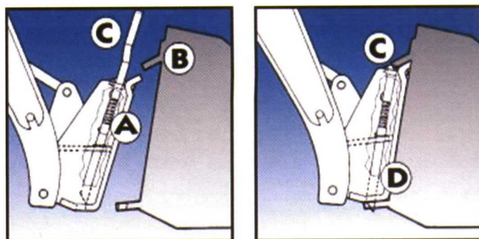
Figura 4. Esquema del sistema estandarizado de acople de implementos al brazo de la máquina.
