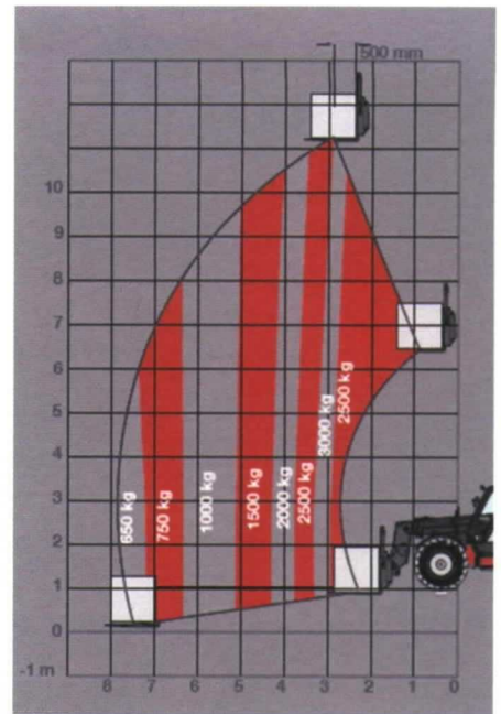
Figura 2. Diagrama representativo de la capacidad de carga de MF 89410. Fuente. www.masseyferguson.com
