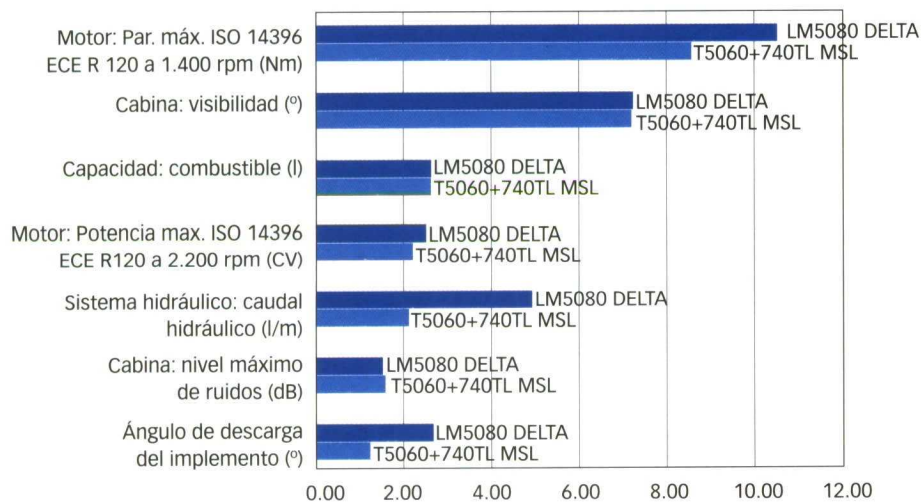
Figuras 5 y 6. Manipulador telescópico New Holland LM5080 Delta frente a New Holland T5060 equipado con cargador frontal New Holland 740TL MSL. Fuente: Elaboración propia a partir de catálogos de New Holland.
