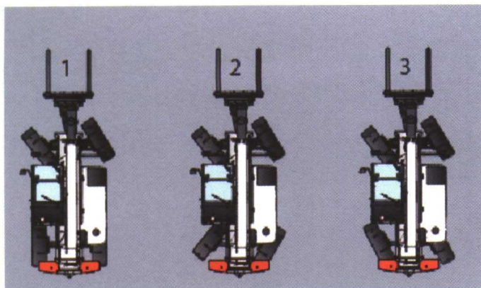
Figura 3. Modalidades de dirección en telescópicas de Bobcat. Fuente. www.bobcat.eu
