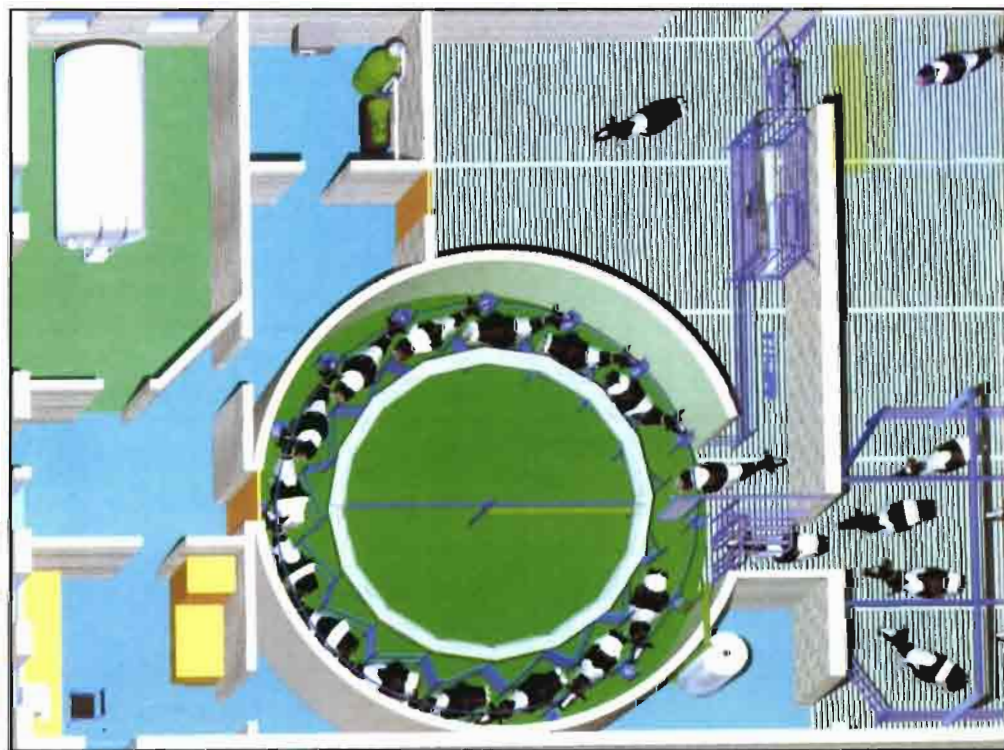
Sala de ordeño rotativa espinas de pescado (Westfalia Separator).
