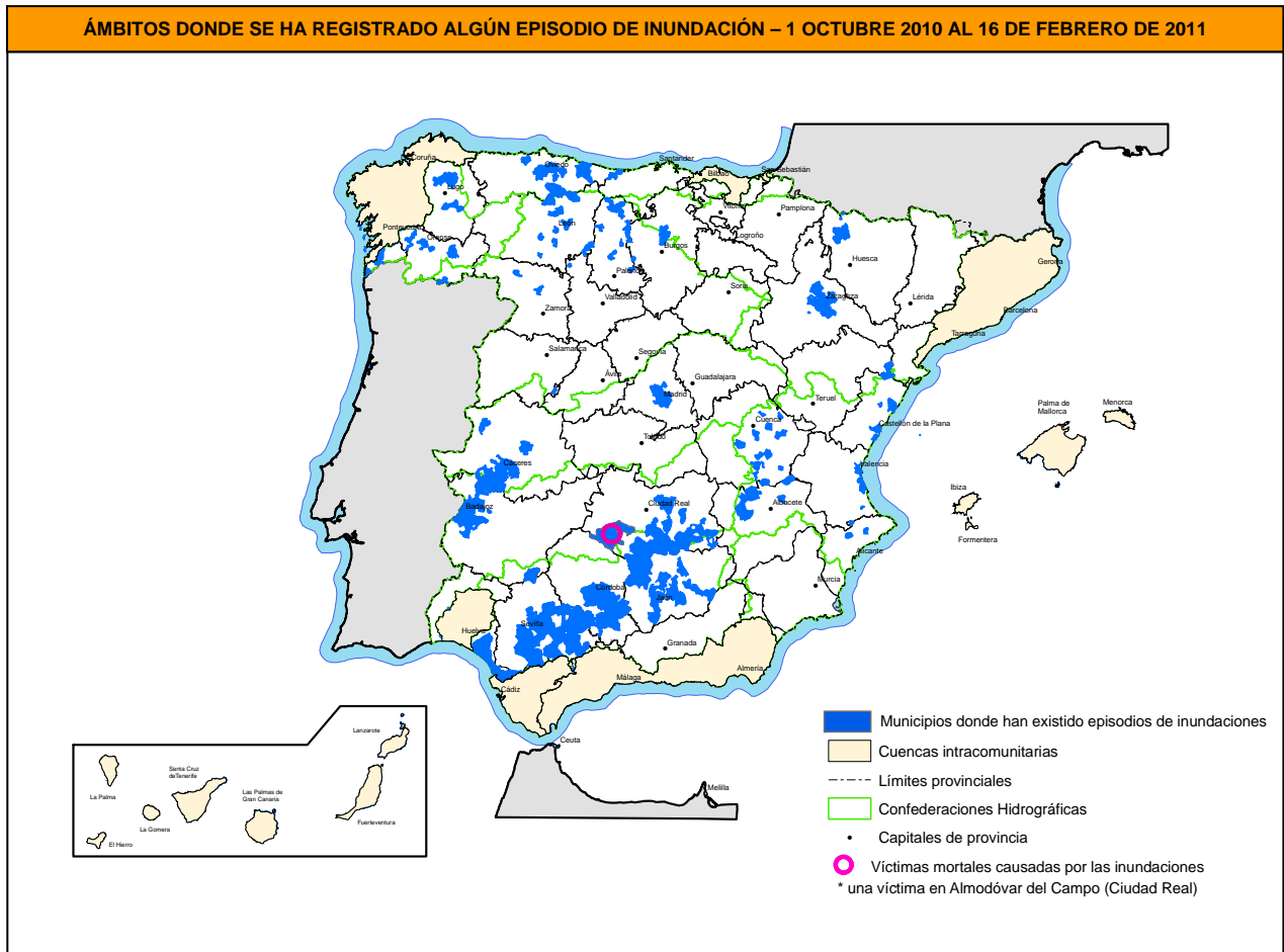
Figura 1. Localización de los episodios de inundaciones – (del 1 octubre 2010 al 16 de febrero de 2011) (Fuente: MARM y Protección Civil)
