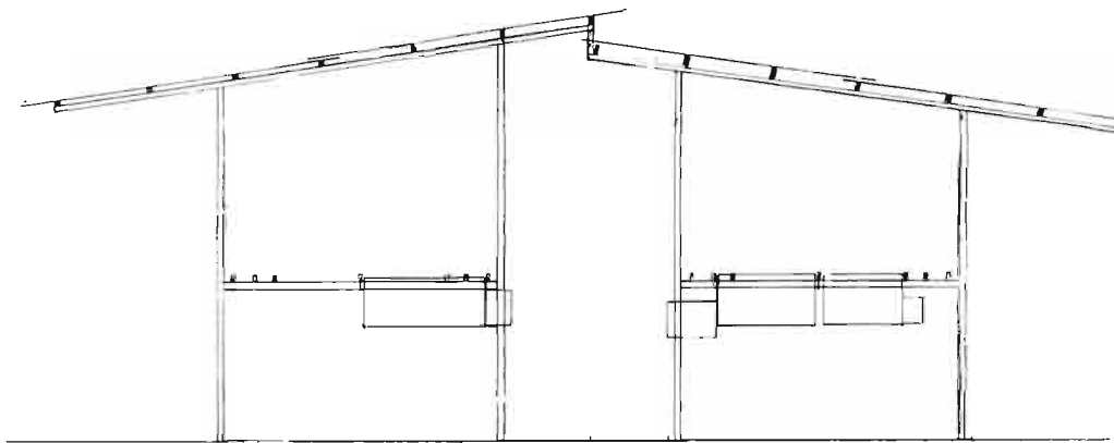
Fig. 2.— Sistema protegido semi aire libre, con dos vertientes de fibrocemento y soportes de metal.
