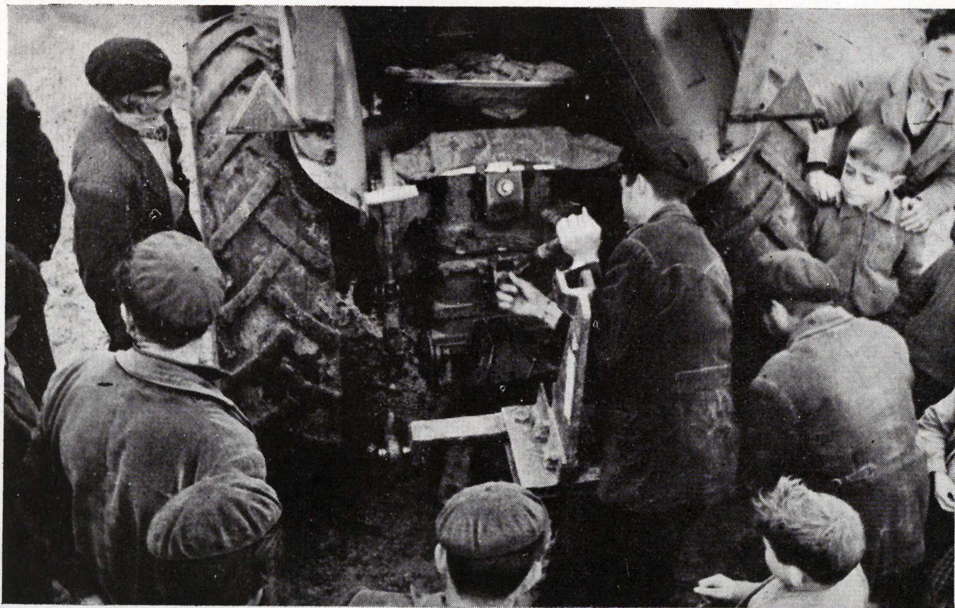
Peñaranda.—Demostración de maquinaria en Macotera. Acoplamiento de un subsolador al tractor.
