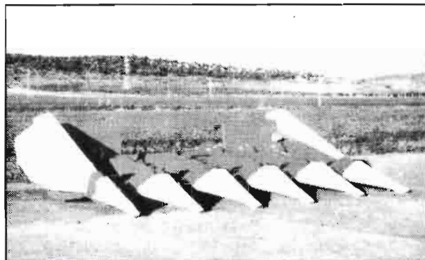
Equipo de corte para girasol.
