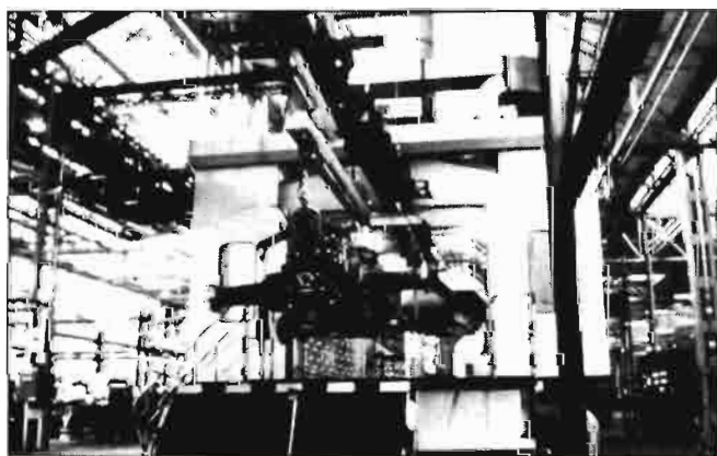
Entrada en la cabina de pintura en la fábrica de Cuatro Vientos.
