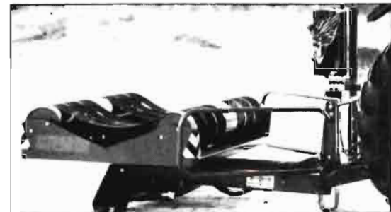
Plastificador de placas cilíndricas Kverneland "Silawrap".
