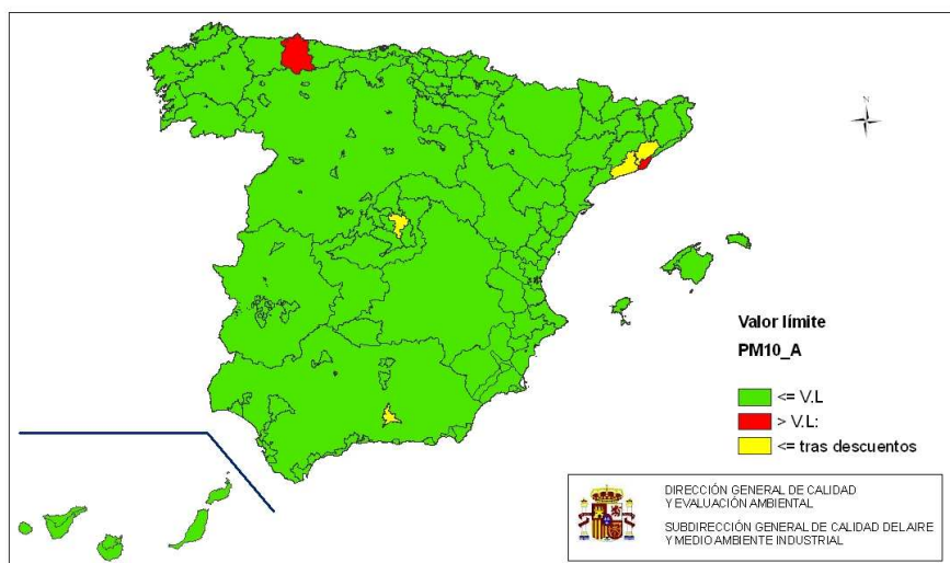
Evaluación de PM10 Datos 2009 Valor límite anual para la protección de la salud tras descuento de intrusiones
