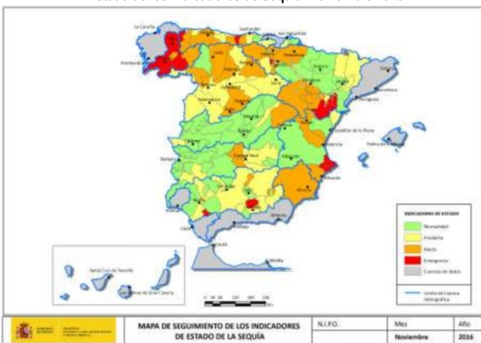
Estado de los Indicadores de Sequía. Noviembre 2016
